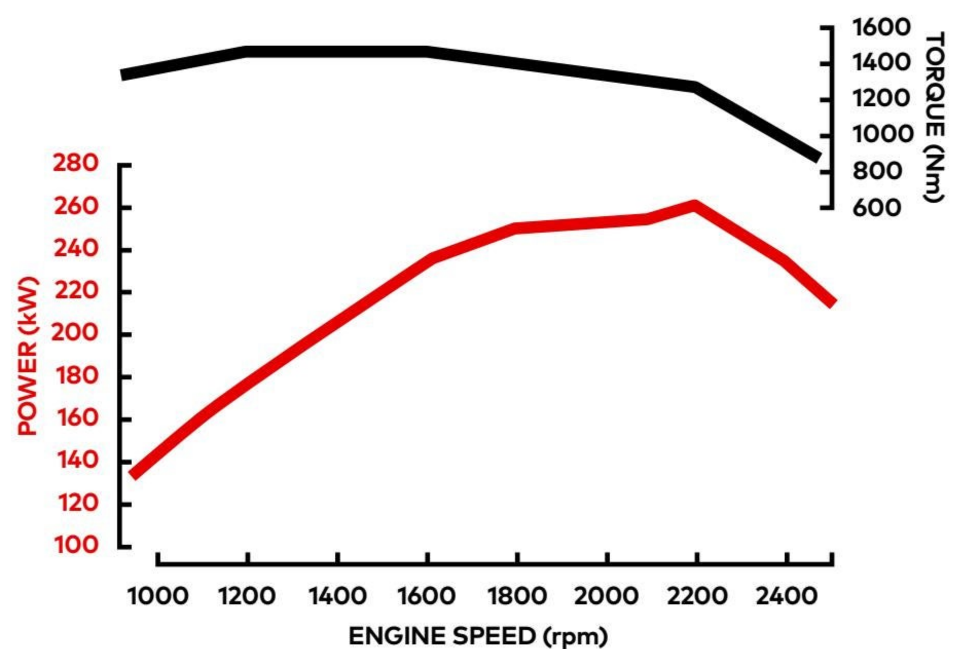
360hp/1400Nm
